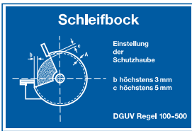
Schleifbock Einstellung der Schutzhaube
